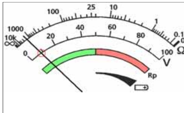
Figura 21: indicación de voltaje de ruido de fondo
