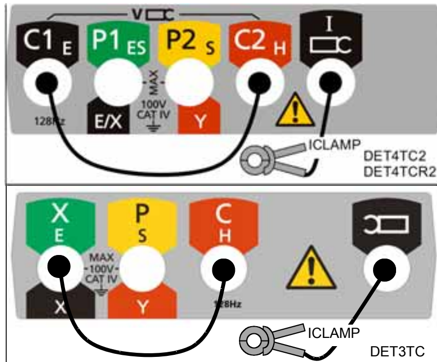
Figura 37: calibración a cero del ICLAMP
