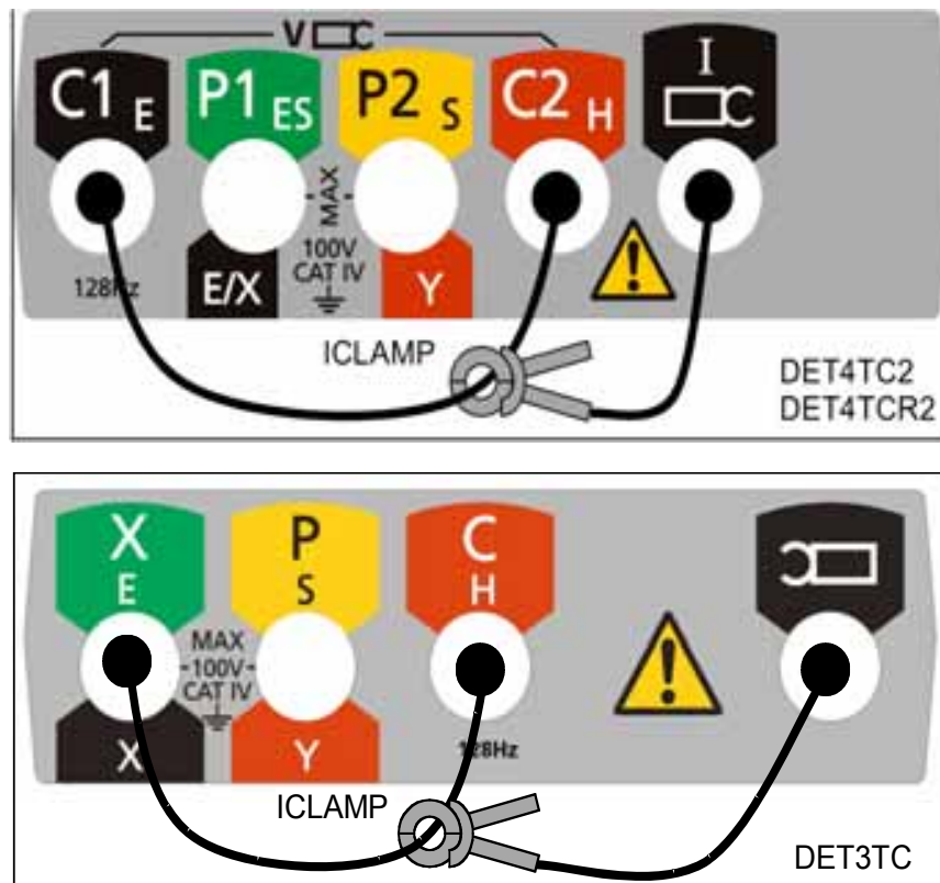
Figura 38: calibración al 100% del ICLAMP
